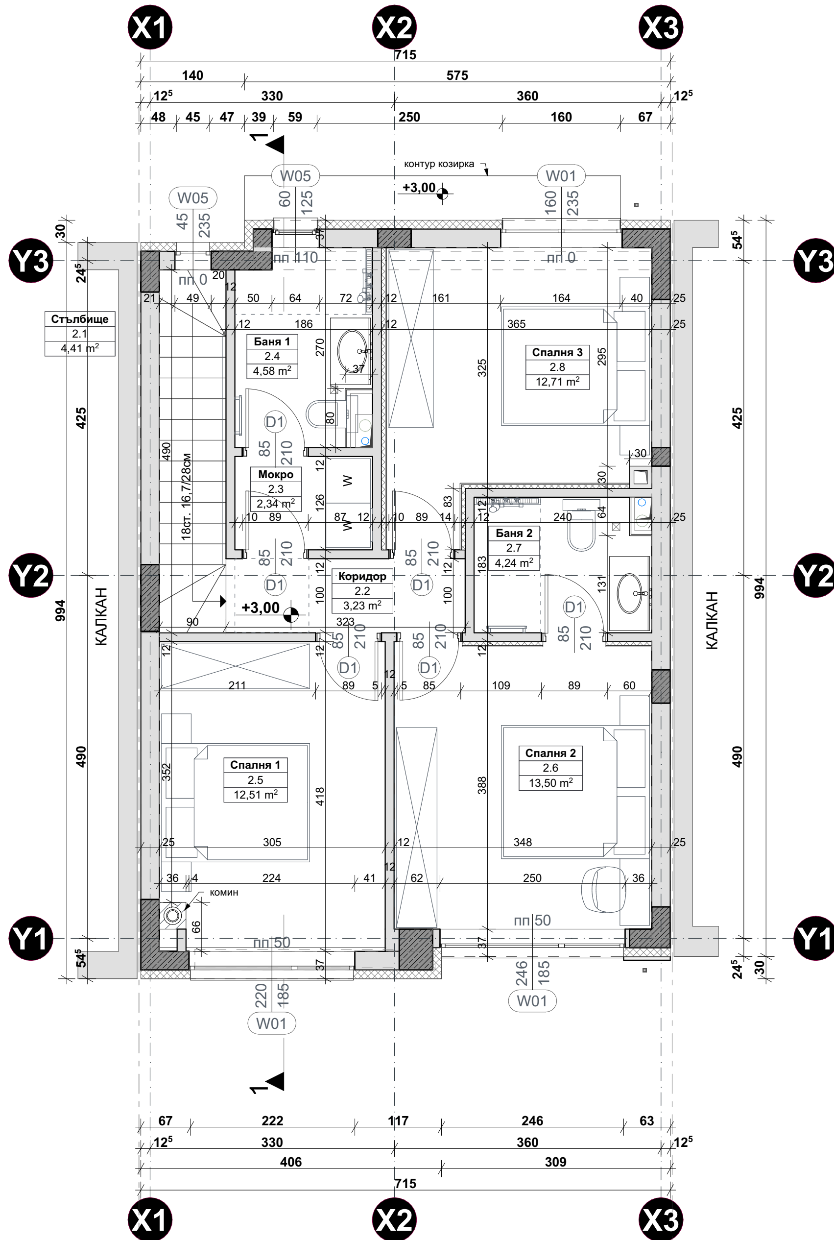
ПЛОЩИ НА КОТА +3,00
